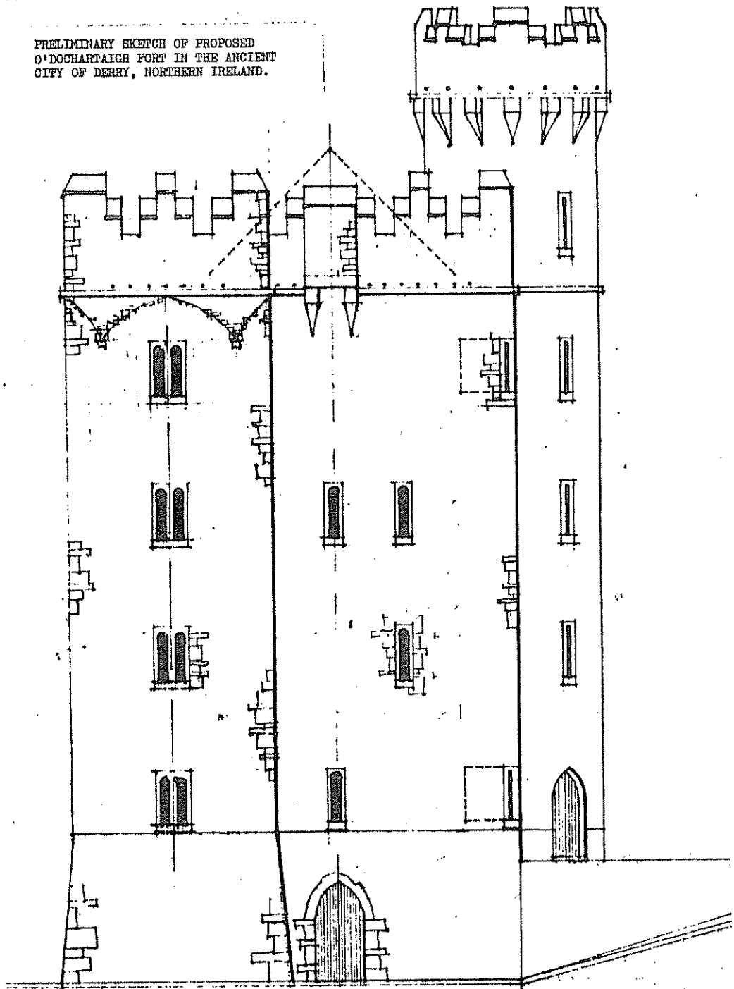
ELEVATION
